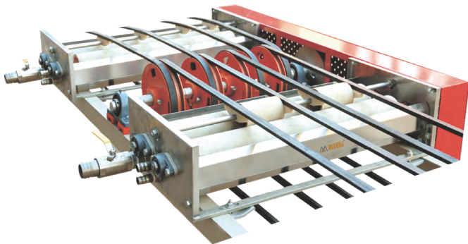
平台底浆机 Engobing Unit (Roller Table Type)
